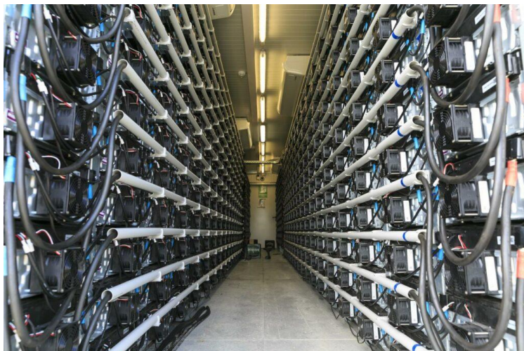
Figura 2.2. Almacenamiento de electricidad en baterías.
