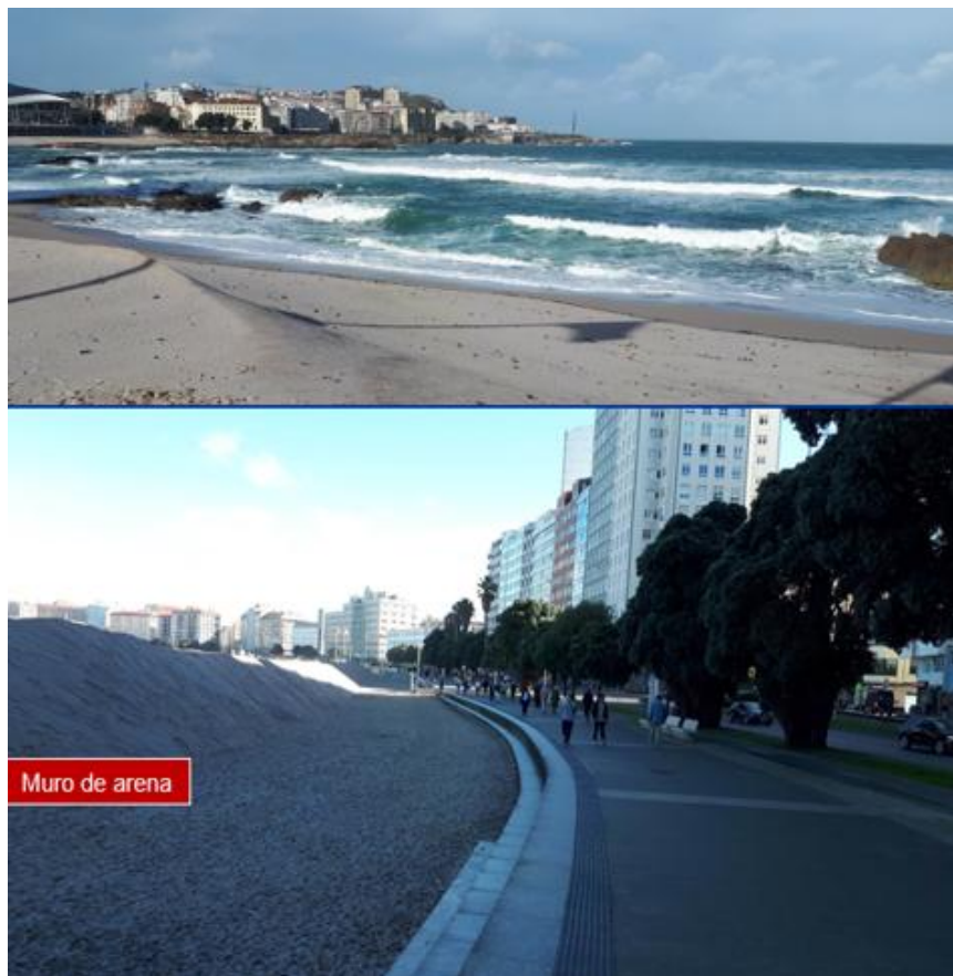
Figura 2.29. Muro de arena para que el fuerte oleaje no atravesase la calle que está enfrente.
